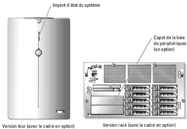
Figure 1-1. Montages de type rack et tour
